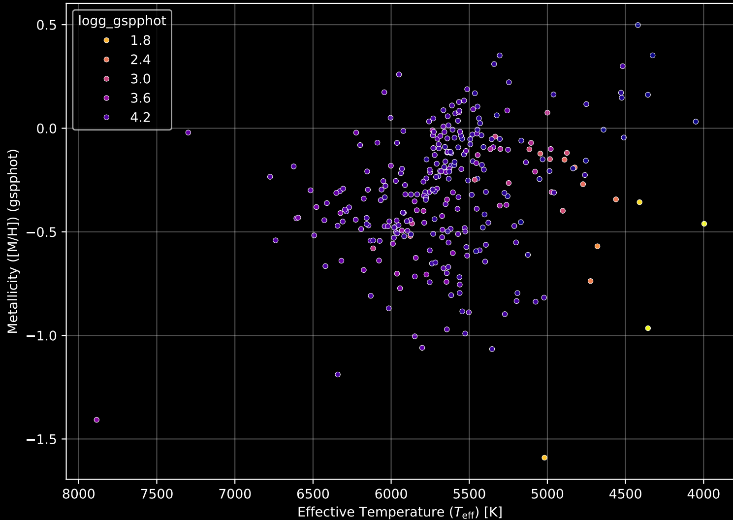
GALAH DR4 Field: [182] Stellar Population Parameters (n= 295)
