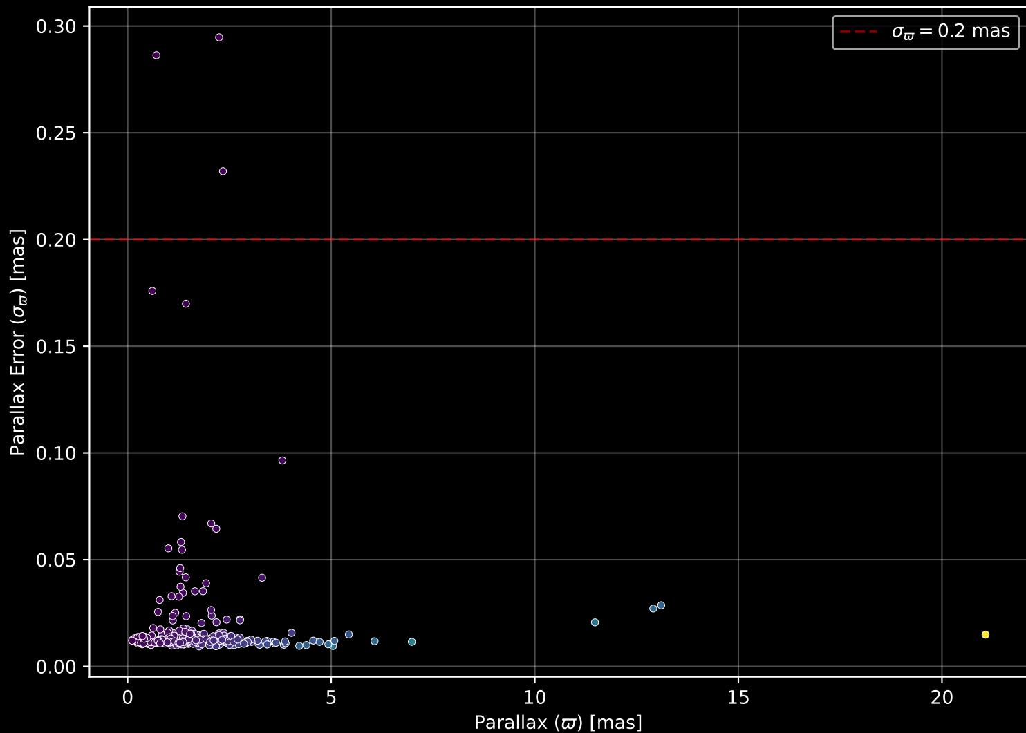
GALAH DR4 Field: [182] Parallax Quality (n= 295)
