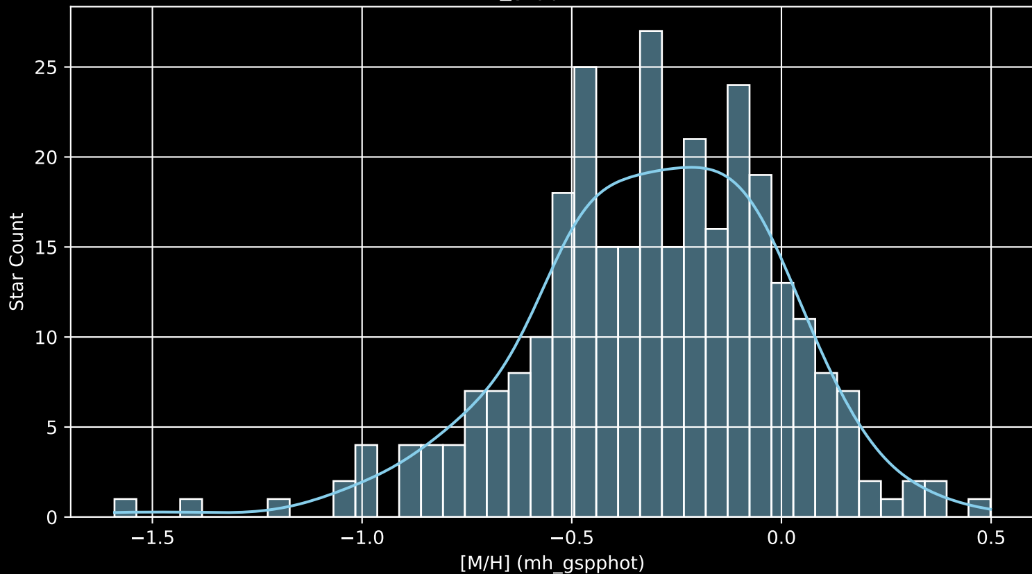
GALAH DR4 Field: [182] [M/H] (mh_gspphot) (n= 295)
